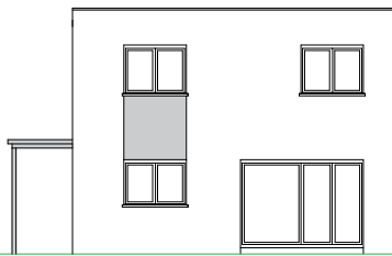
ansicht süd
